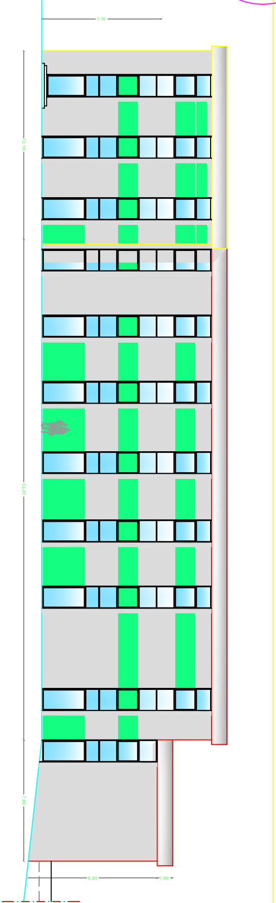
PROSPETTO SU G.R.A. ANTE OPERAM
